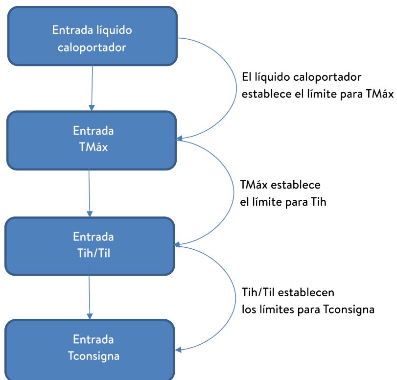
Fig. 23: Secuencia de las entradas
