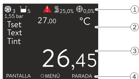
Fig. 26: Ventana básica con barra de estado y barra de softkeys
