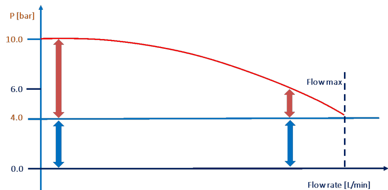
Fig. 55: Diagrama de presión del sistema
