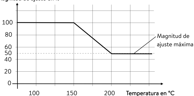
Fig. 47: Limitación dinámica de la potencia calorífica
