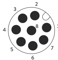
Fig. 12: Asignación de clavijas de la interfaz Safety
