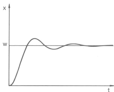
Fig. 81: Parámetros de regulación T_n y T_v demasiado bajos
