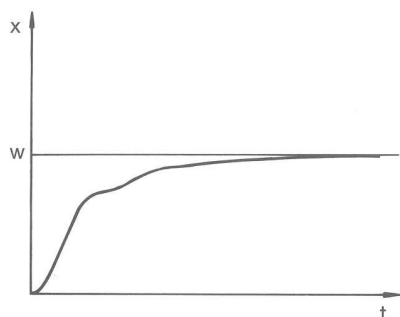
Fig. 82: Parámetros de regulación T_n y T_v demasiado altos
