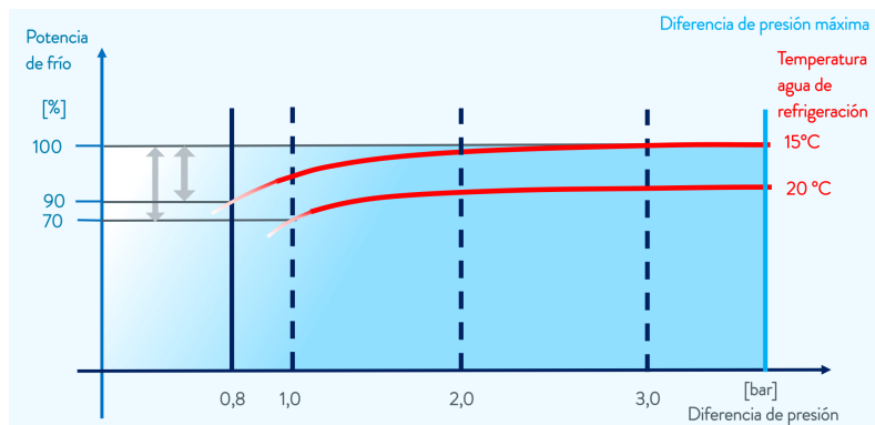
Fig. 99: Diferencia de presión del agua de refrigeración
