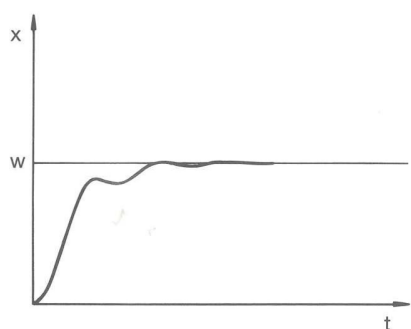
Fig. 80: Parámetro de regulación X_p demasiado bajo
