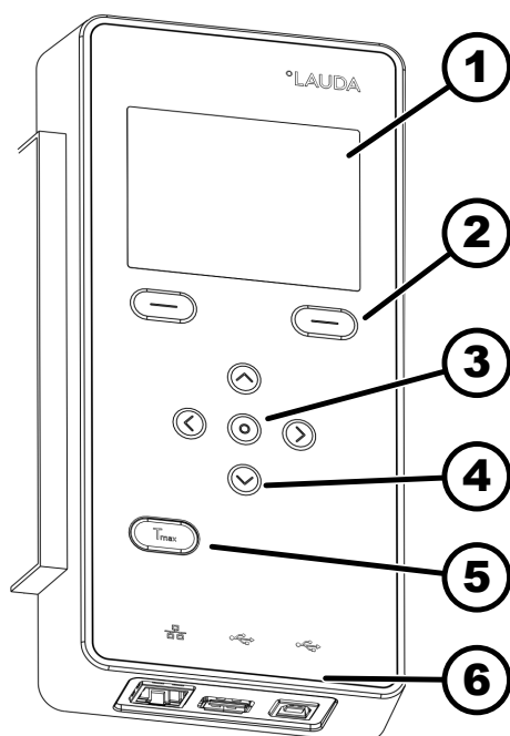
Fig. 28: Unidad de mando
