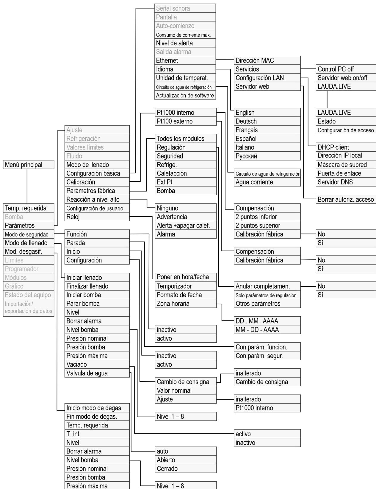
Fig. 38: Menú, parte 2, continúa de la página anterior
