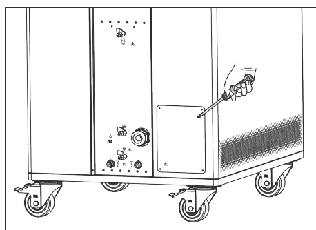
Fig. 20: Chapa de revestimiento aguas arriba de la caja de conexiones
