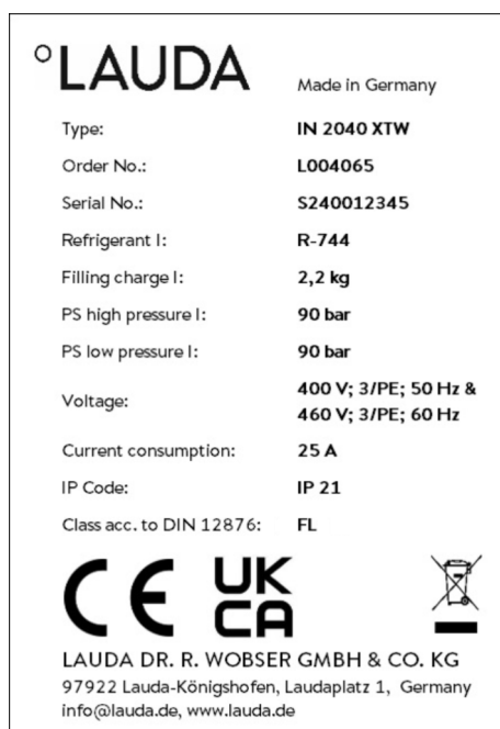
Fig. 10: Placa de características (ejemplo)
