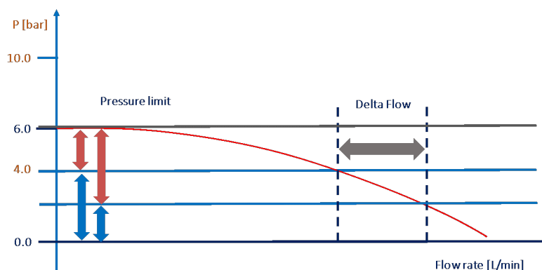
Fig. 56: Diagrama de presión del sistema
