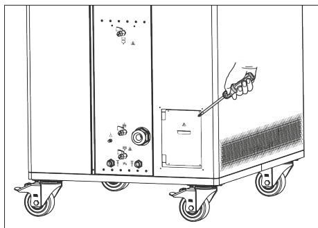
Fig. 21: Tapa de la caja de conexiones
